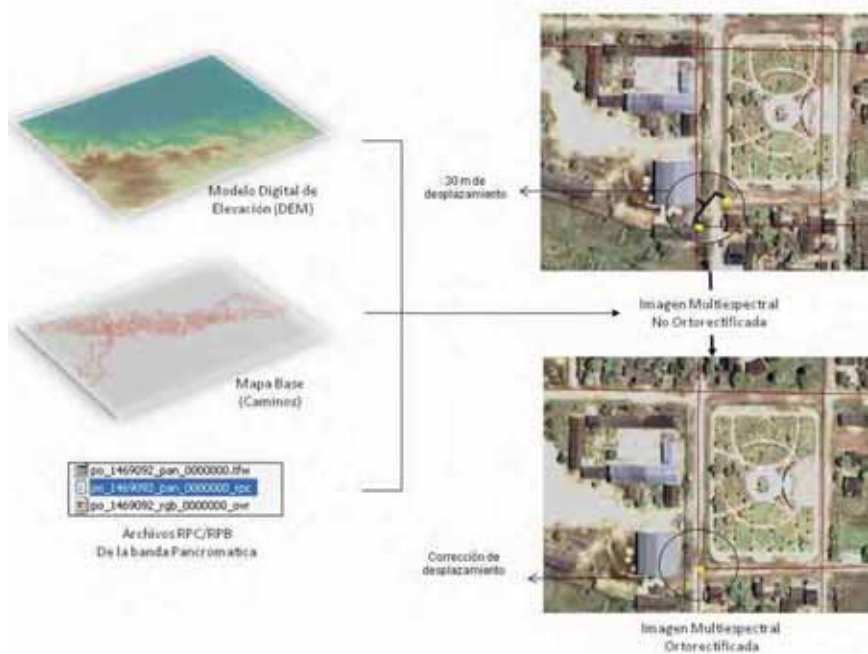
Figura 42. Corrección geométrica
